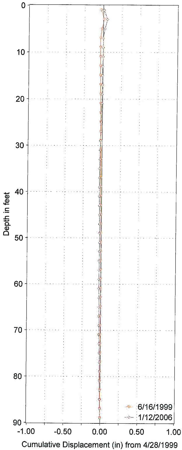
99448 B-2, A-Axis
