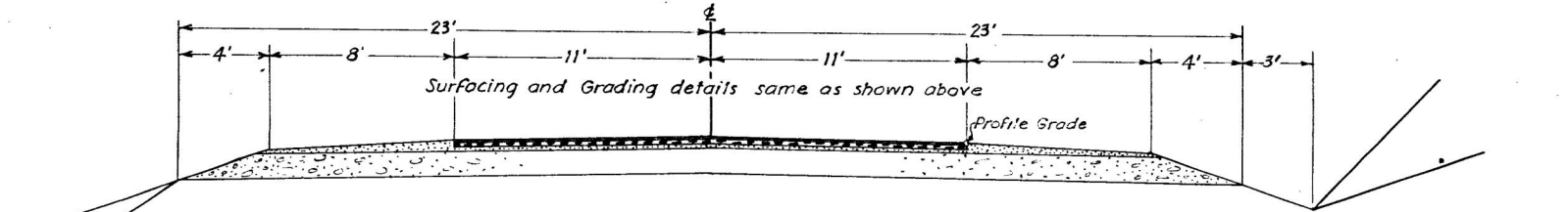
Grading and Paving Section Sta. 476+50 to Sta. 479+50 Sta. 491+50 to Sta. 494 Sta. 514 to Sta. 519+31.7
