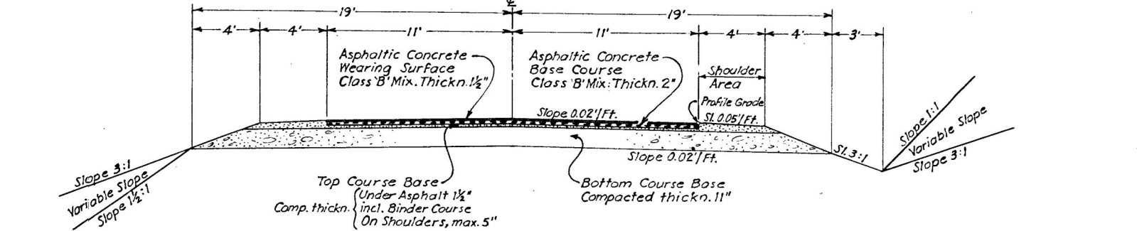
Grading and Paving Section Sta. 431 to Sta. 433+50 Sta. 438+50 to Sta. 442+50 Sta. 454+50 to Sta. 457
